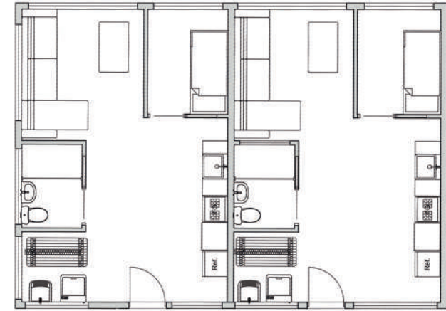
Plantas UH (35m²) 1:50
