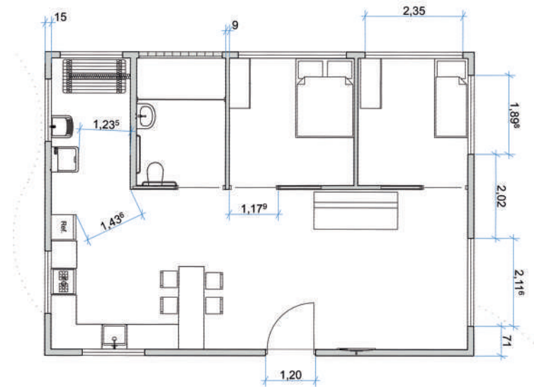
Planta Unidades PCD (70m²) 1:50
