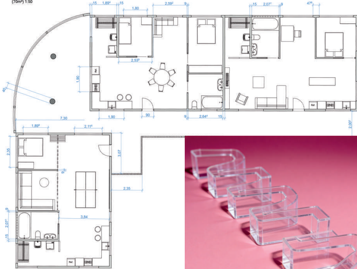
Planta Unidades Habitacionais Tipo 1, 2 e 3 (70m²) 1:50
